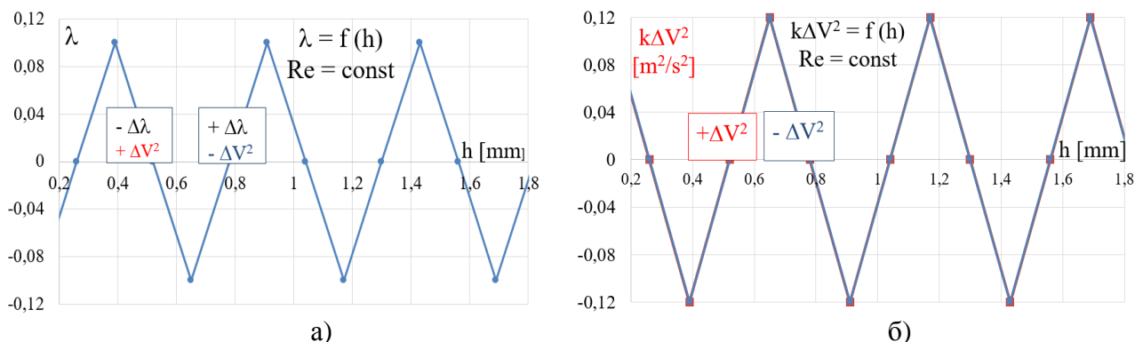
Рис. 3. Зміна коефіцієнта гідравлічного тертя та динамічної складової енергії потоку при лінійній зміні висоти каналів при Re = 1700 : а – залежність \lambda = f(h) при Re = 1700 ; б – залежність k\Delta V^2 = f(h) при Re = 1700
